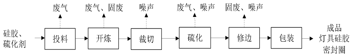
图 2-2 灯具硅胶密封圈生产工艺流程及产污环节图
